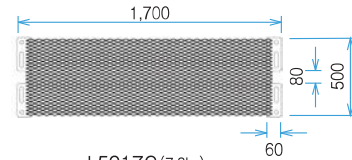
L5017G (7.8kg) HPFスキマ板17
