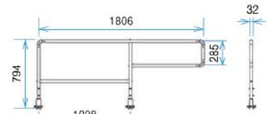
SPカイドン手摺 (4.2kg) (VKTSP)
