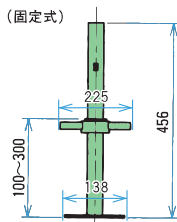
N37×450G (5.8kg) (N3745)
