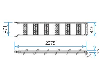
SPカイドン (10.5kg) (VKSP)
