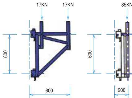
BK6G (9.3kg) HPFブラケットBK6
