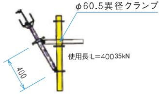
HHS4P (2.8kg) HPFハンチサポート
