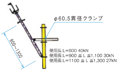
HHS813P (6.0kg) HPF伸縮ハンチサポート
