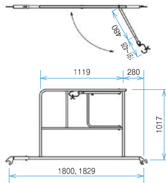
SPセーフティガード (12.0kg) (ASGSP)
