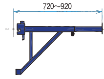
BKSS0609G (5.0kg) (LBK609G)
