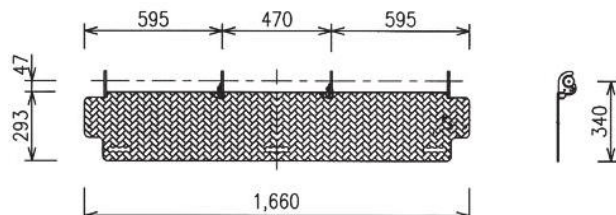
SK18 (15.0kg) すき間ステップ18
