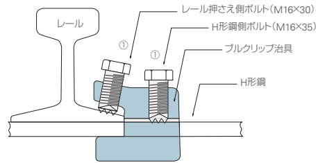
適用レール: 15kg~30kg 適用H鋼製枕木: フランジ厚6~9mm
