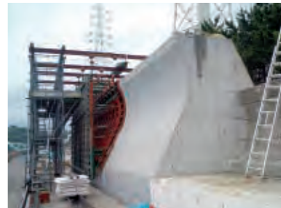
防潮堤
