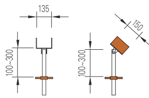
HPF 自在大引受けジャッキ (PF-ONF35×450P) (5.8kg)
