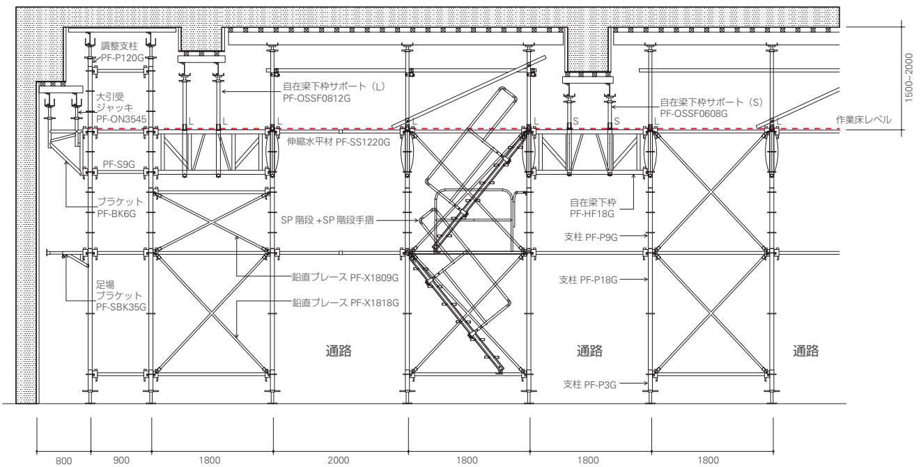
参考図面例
