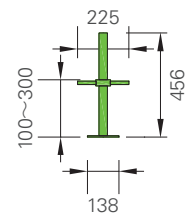
HPF ジャッキベース (PF-N37×450G) (5.8kg)
