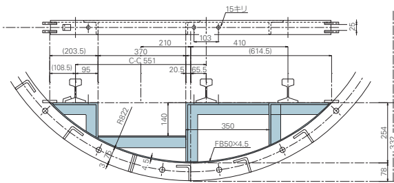
アングル製の1,800ミリ用
