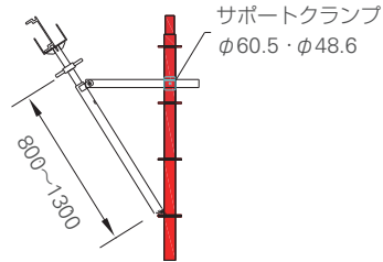
HPF 伸縮ハンチサポート (PF-HHSS813P) (6.0kg)
