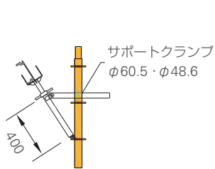
HPF ハンチサポート (PF-HHS4P) (2.8kg)
