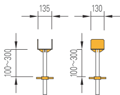
HPF 大引受けジャッキ (PF-ON35×450P) (5.5kg)
