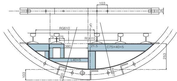
アングル製の2,000ミリ用
