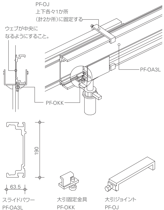
アルミ大引シングル(単純梁)使用時
