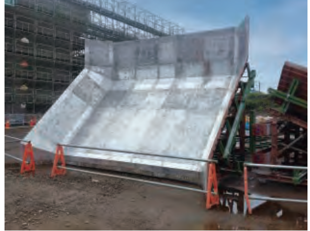
45°梁底型枠
