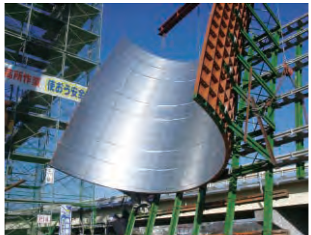
大口径円形梁底
