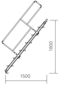
SP 階段 (VKSP) (10.5kg) SP 階段手すり (VKTSP) (4.2kg)
