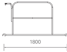
SPセーフティガード (ASGSP) (12.0kg)
