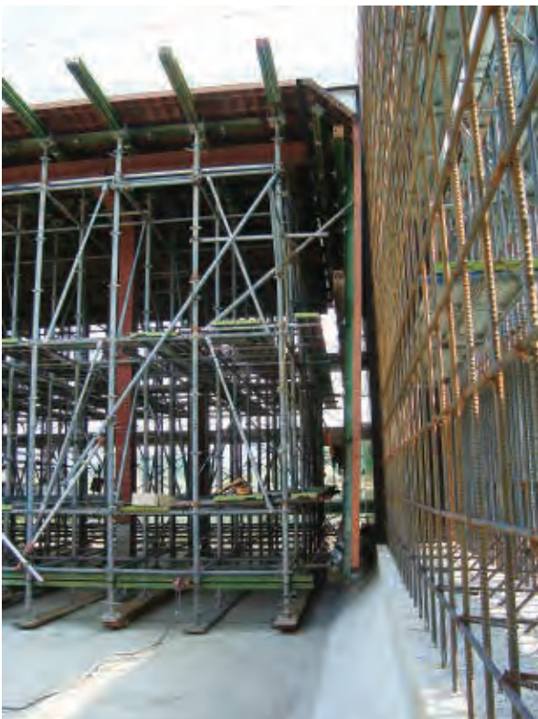
移動台車 支保工 + 型枠 (スラブ側面)
