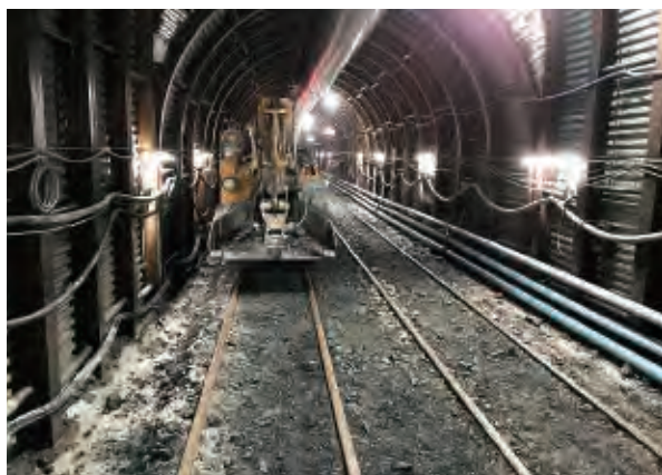
NATM レール工法
