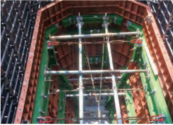
中空型枠 内ハンチ
