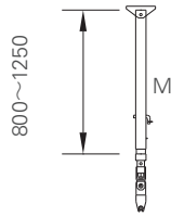
HPF 大引サポート M (PF-OSSF0812P) (4.7kg)
